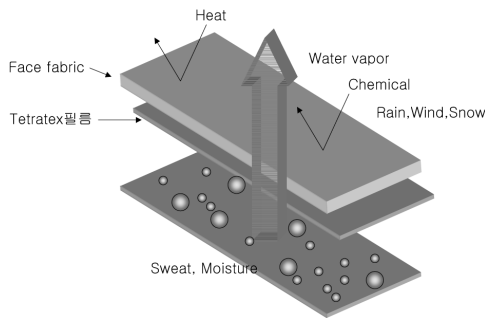
Figure 13. 테트라텍스 구조도.
